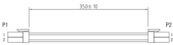
外形図
