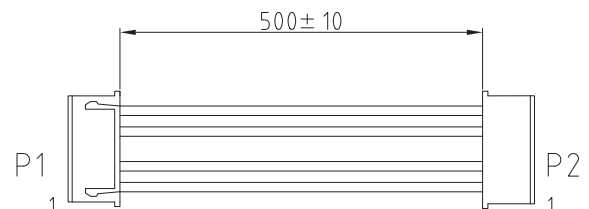
外形図
