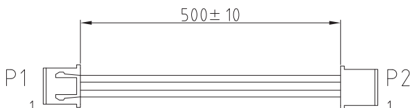
外形図
