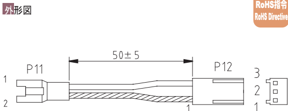
外形図
