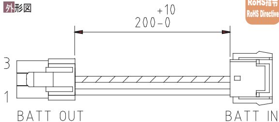
外形図
