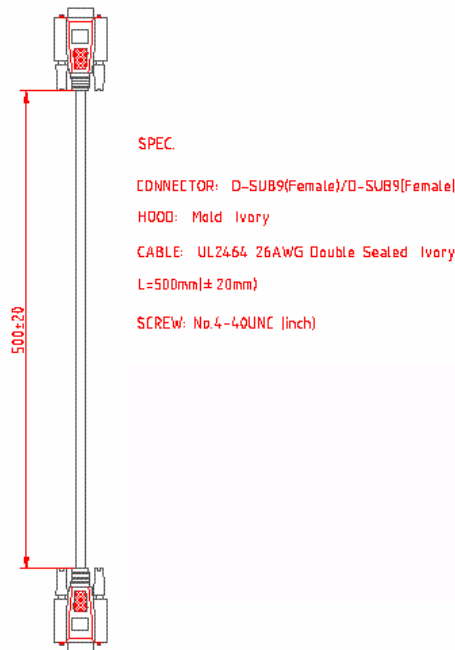
図 6.14 接続ケーブル
