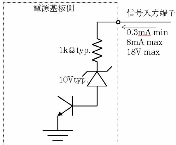
図 6.10 FAN C 信号入力
