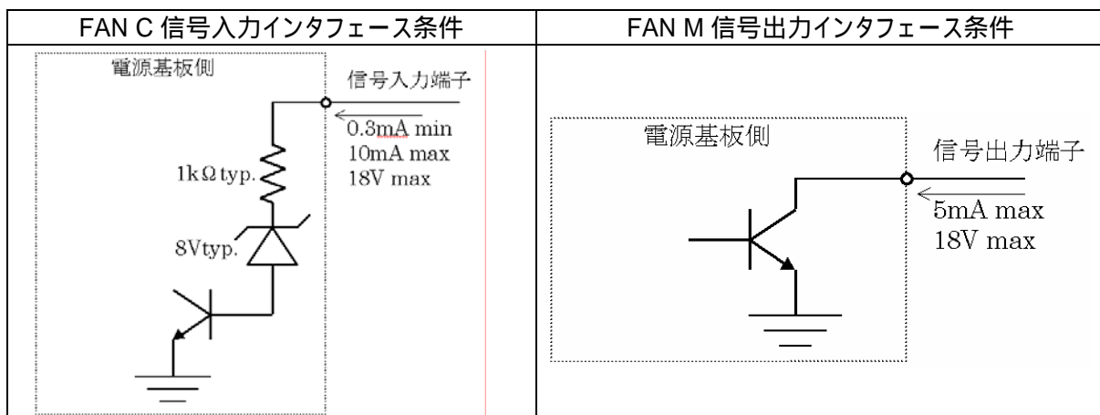
図 6.9 FAN C 信号入力、FAN M 信号出力
