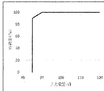
図4. 低入力電圧ディレーティング
