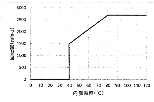
図5. ファンモータ変速回転数 (目安)
