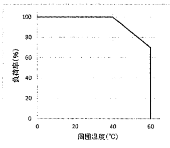
図3. 温度ディレーティング
