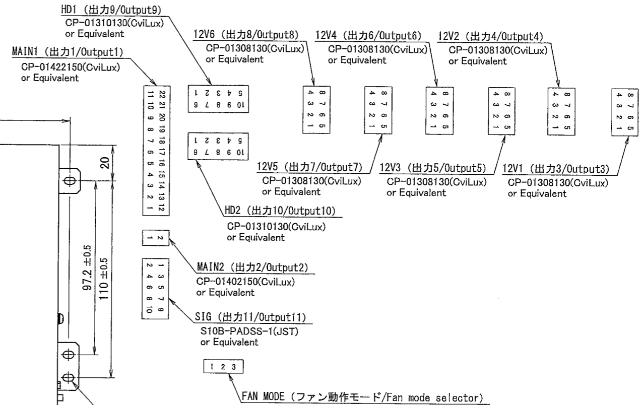
ピン配置図/Pin Assignment
