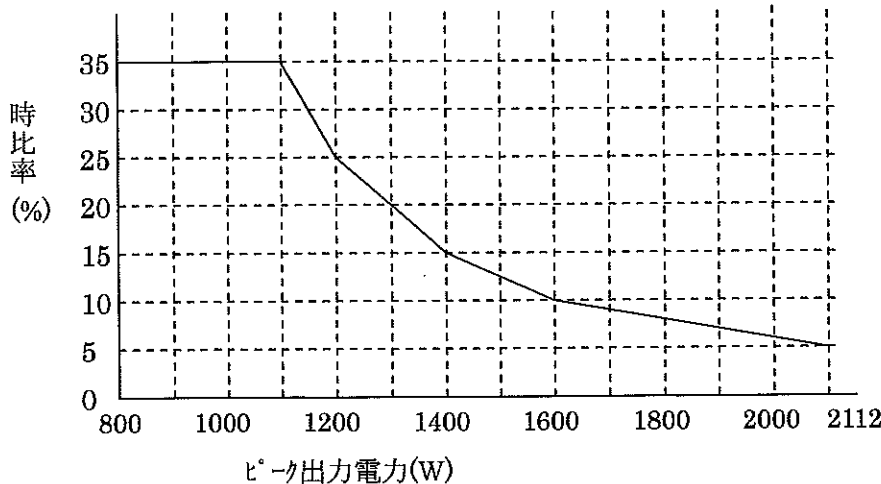
時比率VSピーク出力電力表
