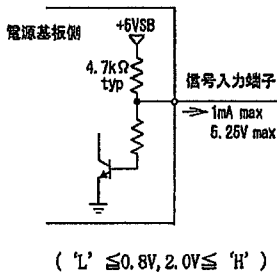
PS_ON 信号入力回路
