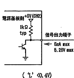
PWR_OK 信号出力回路
