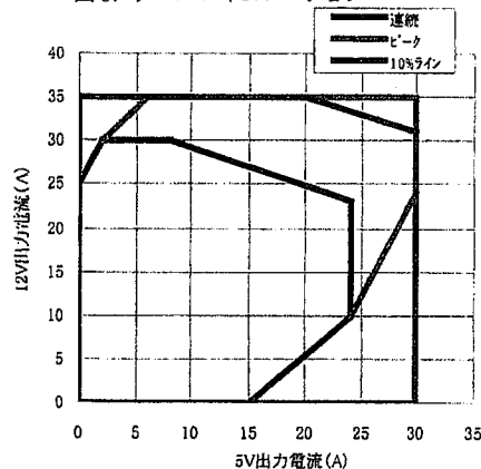
図5. クロスレギュレーション
