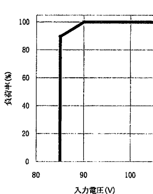
図4. 低入力電圧ディレーティング
