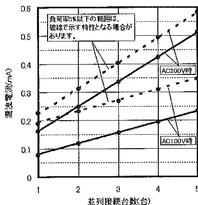
並列接続数と漏洩電流(typ)
