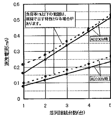
並列接続数と漏洩電流(typ)
