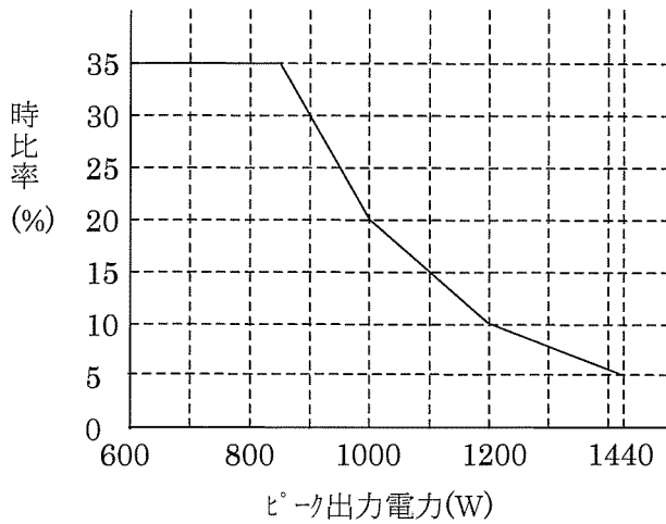
時比率VSPeak出力電力表
