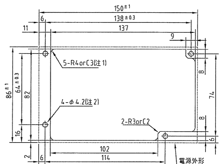
推奨電源取り付け穴加工図
