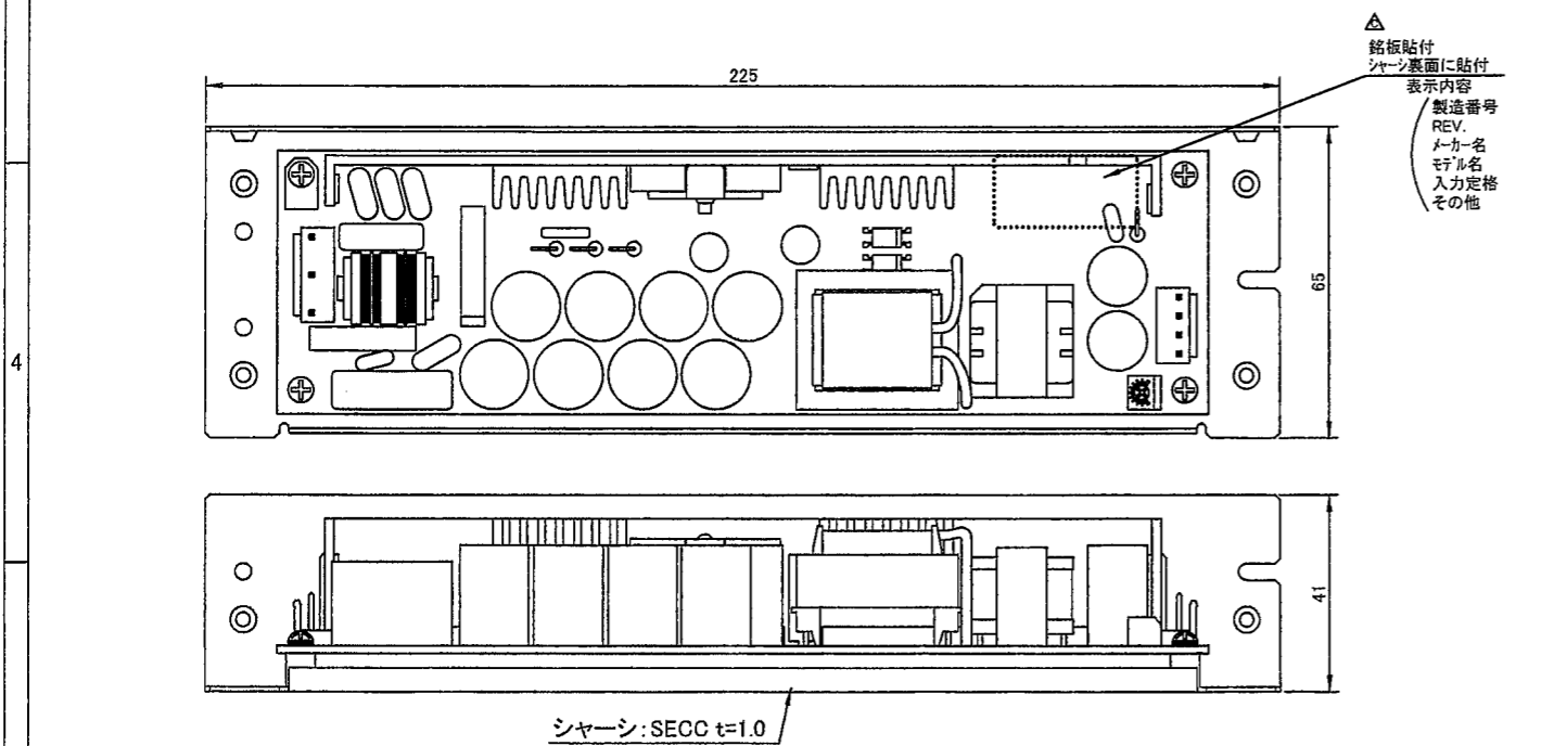
※取付寸法はシャーシ・カバー付きタイプと同じ △ シャーシ付きタイプ 形式: OZ-060-***-*00-C
