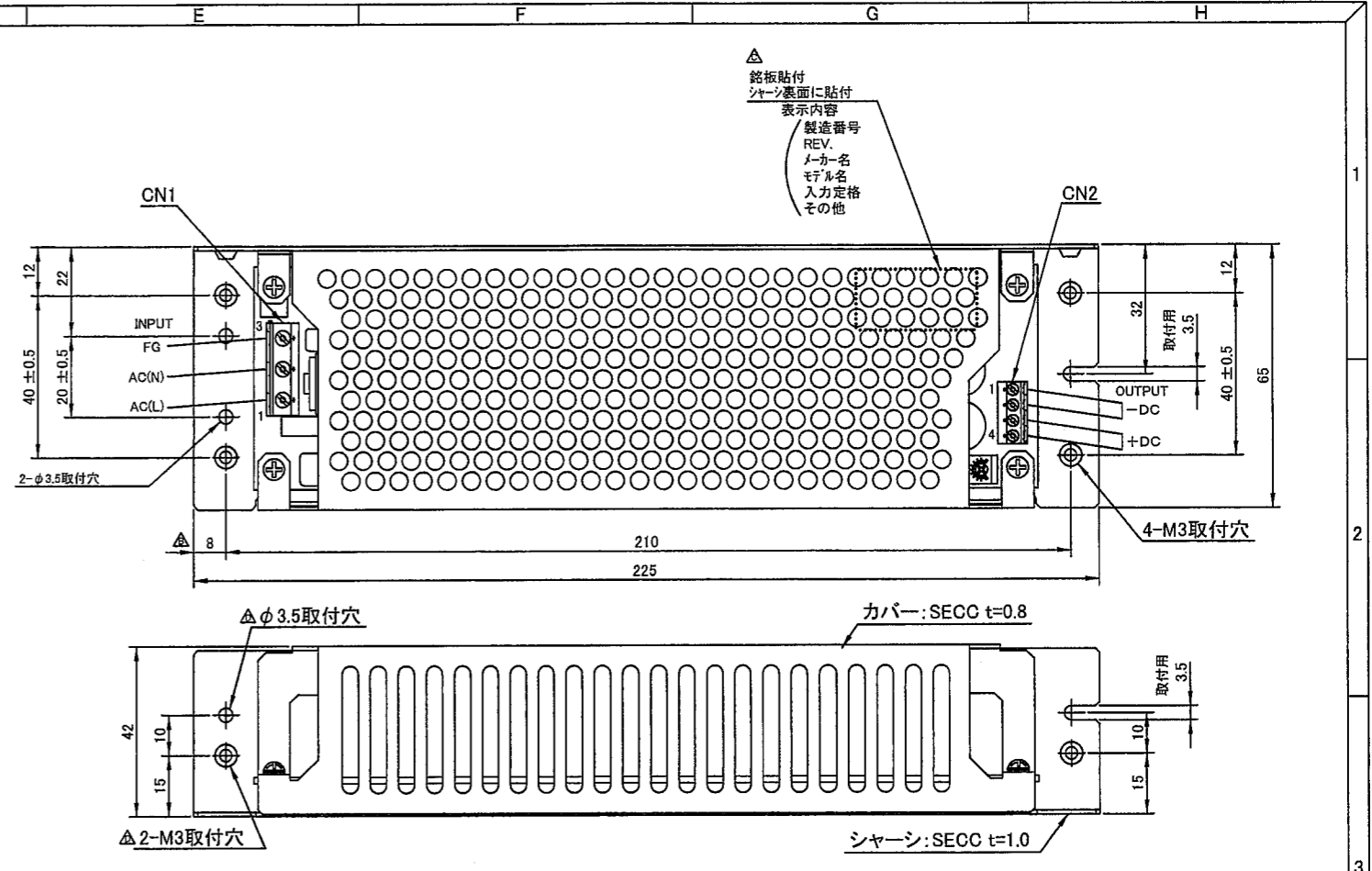
シャーシ・カバー付きタイプ 形式: OZ-060-***-*00-K
