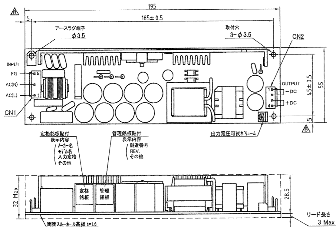
シャーシ・カバー無しタイプ 形式: OZ-060-***-*00
