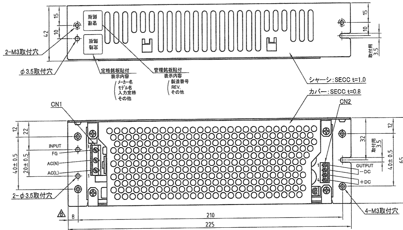
シャーシ・カバー付きタイプ 形式: OZ-060-***-*00-K
