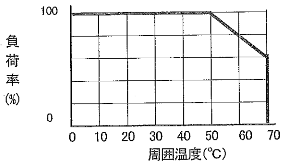
図1. 温度ディレーティング図
