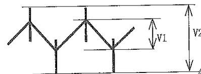
図2. リップル・スパイクの定義
