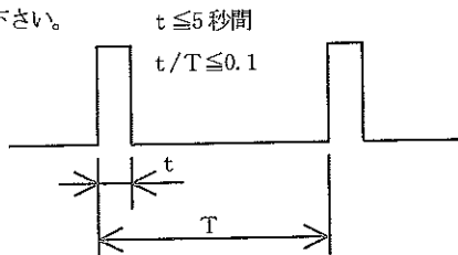
図1. 瞬時最大出力電流・電力の時比率
