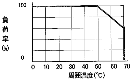
図1. 温度ディレーティング図
