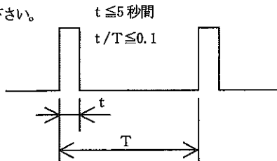
図1. 瞬時最大出力電流・電力の時比率
