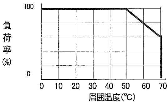
図1. 温度ディレーティング図
