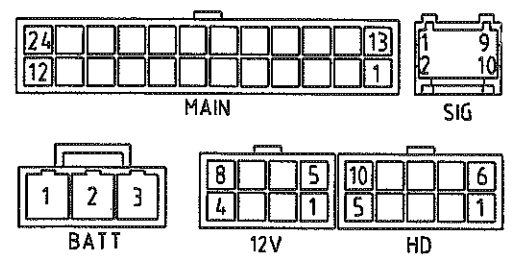
※コネクタのサイン詳細図 ※Pin assignment
