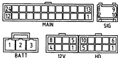
※コネクタのサイン詳細図 ※Pin assignment
