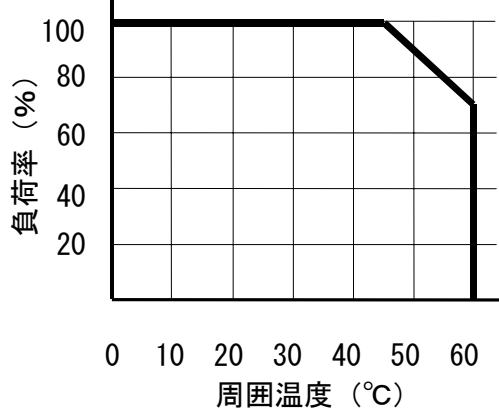
図1 温度ディレーティング図
