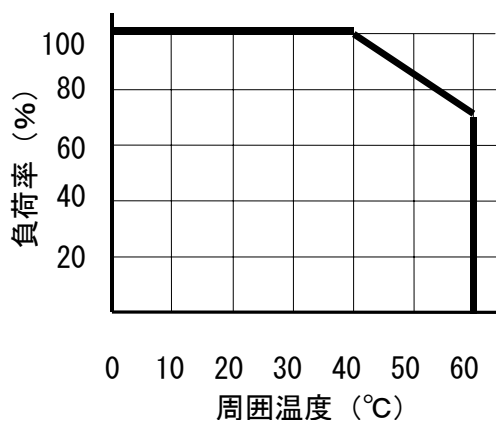
図1 温度デレーティング図
