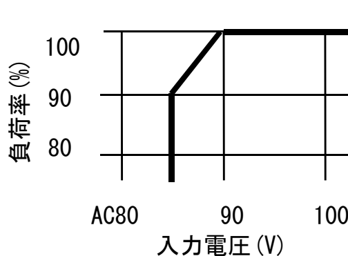
図2 低入力電圧ディレーティング図
