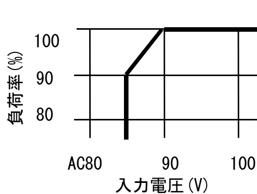
図2 低入力電圧デレーティング図
