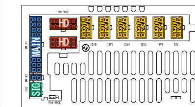
ハーネス接続可能数
