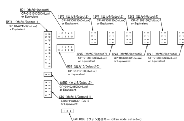
ピン配置図/Pin Assignment
