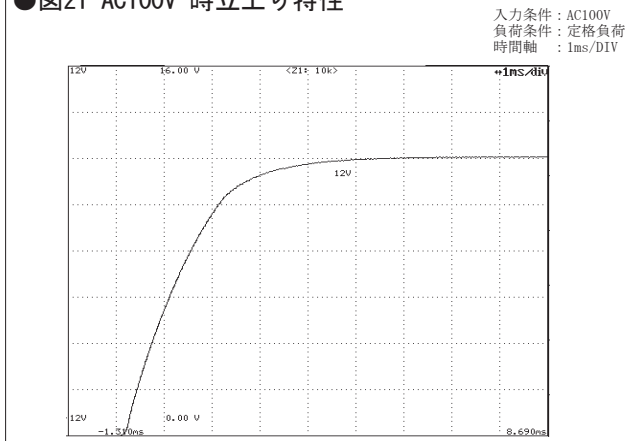
● 図21 AC100V 時立上り特性
