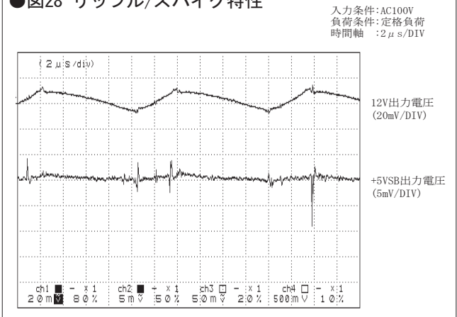
●図28 リップル/スパイク特性
