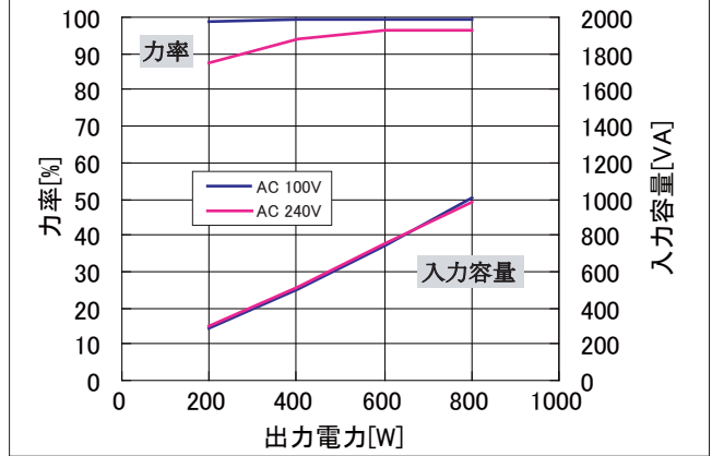
● 図18 力率/入力容量—出力電力特性
