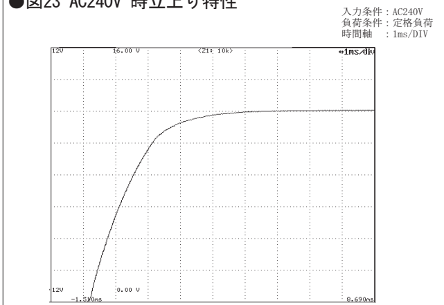
● 図23 AC240V 時立上り特性
