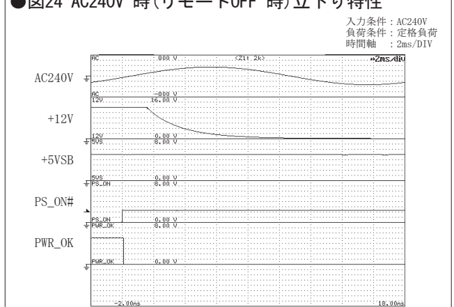
● 図24 AC240V 時(リモートOFF 時) 立下り特性
