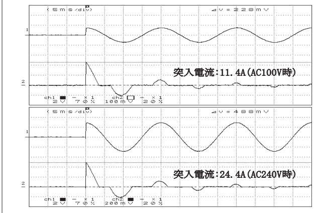
● 図19 突入電流特性
