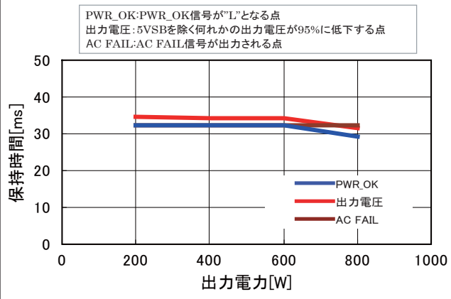
●図25 出力保持時間—出力電力特性
