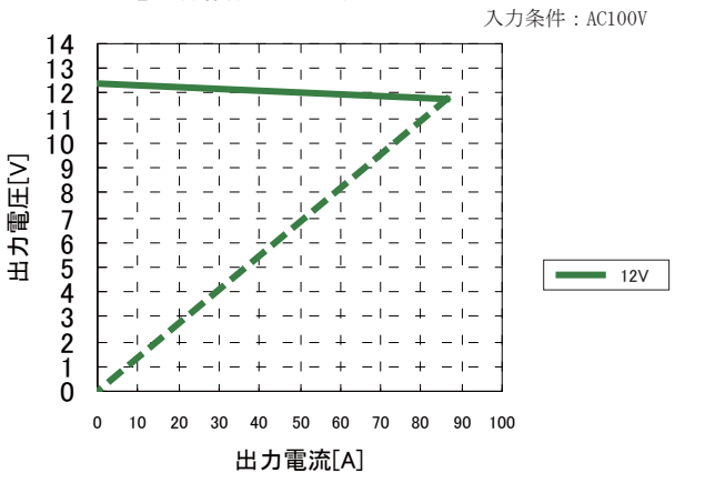
●図29 過電流保護特性 (V-I特性)
