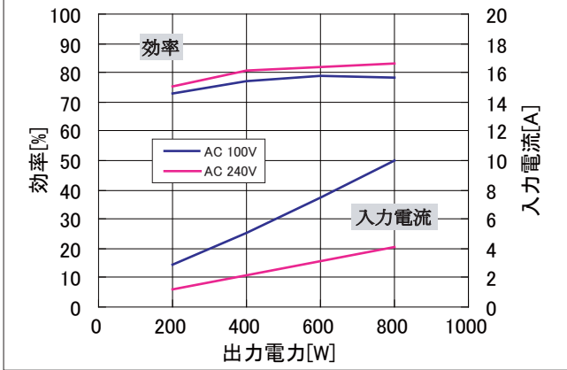
● 図17 効率/入力電流—出力電力特性
