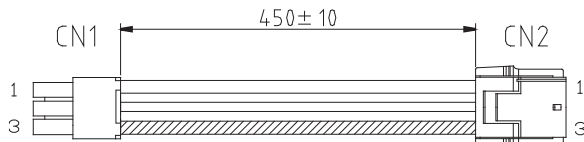
外形図
