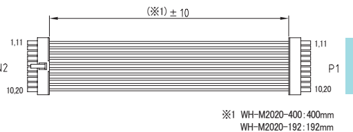
外形図
