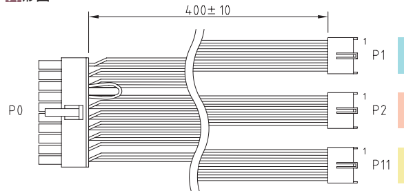
外形図
