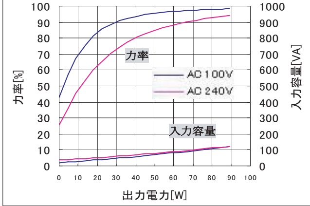
●図6 力率/入力容量-出力電力特性
