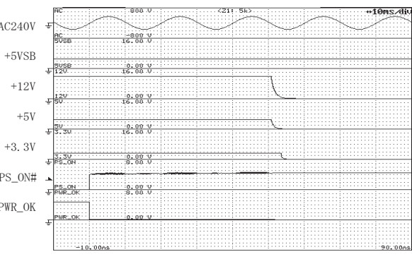
●図12 AC240V 時(リモートOFF 時)立下り特性
