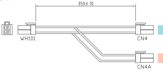
製品仕様
