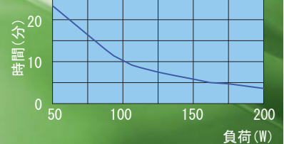
バッテリーパックアップ放電特性 (バッテリーパック使用初期の参考値であり保証値ではありませんのでご注意ください。)
