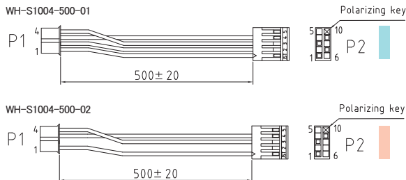
外形図
