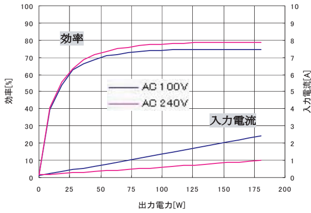
●図20 効率/入力電流—出力電力特性
