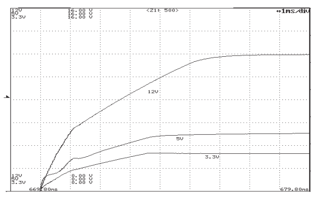
●図26 AC100V 時立上り特性
