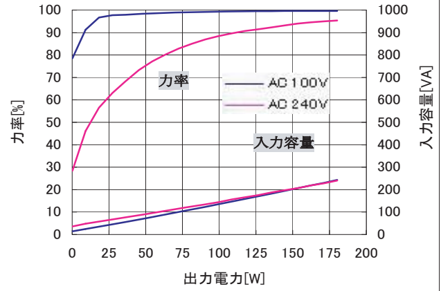
●図21 力率/入力容量—出力電力特性
