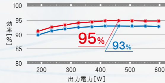
効率グラフ (UZP-600-A24、実測の一例)
