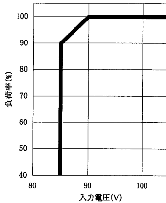
図4. 低入力電圧ディレーティング
