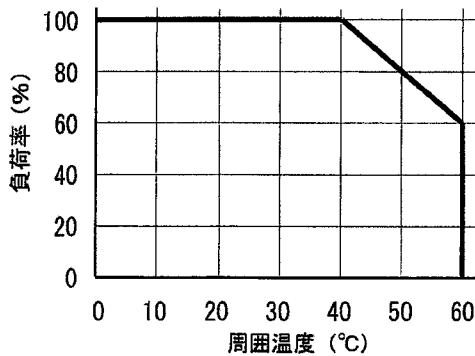
図1. 出力電流・電力デレティング表
