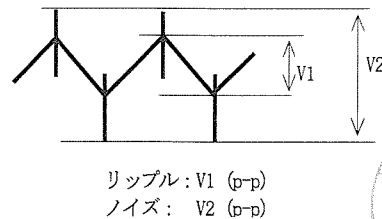
図2. リップル・スパイクの定義
