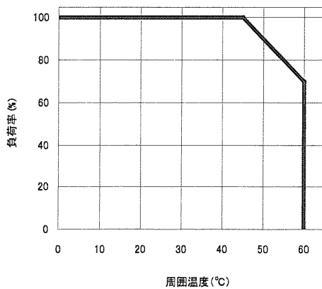
図3. 温度ディレーティング
