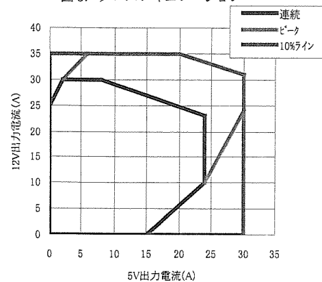
図5. クロスレギュレーション
