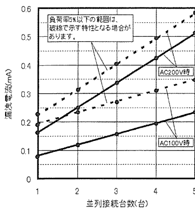
(12V, 15V タイプの漏洩電流) 並列接続数と漏洩電流(typ.)
