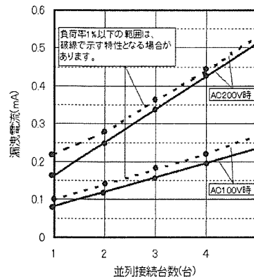
(24V, 36V, 48V タイプの漏洩電流) 並列接続数と漏洩電流(typ.)
