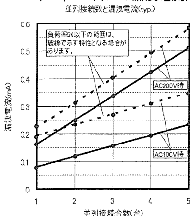
(12V, 15V タイプの漏洩電流)
