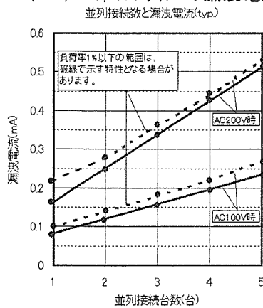
(24V, 36V, 48V タイプの漏洩電流)
