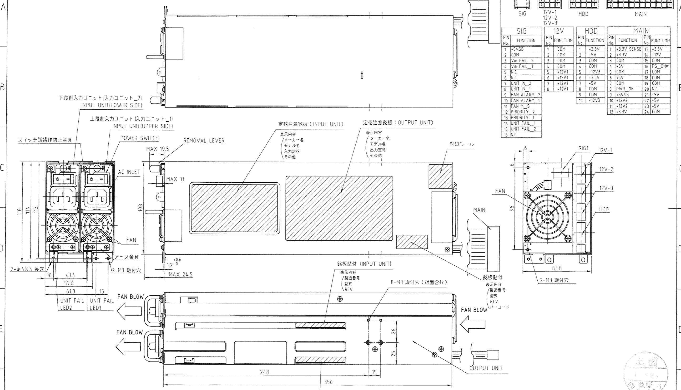
※コネクタピンアサイン詳細図
