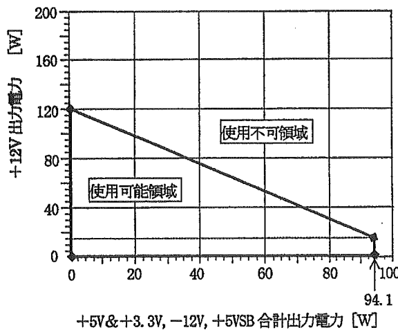
図3. 強制空冷時 (外部ファン使用)
