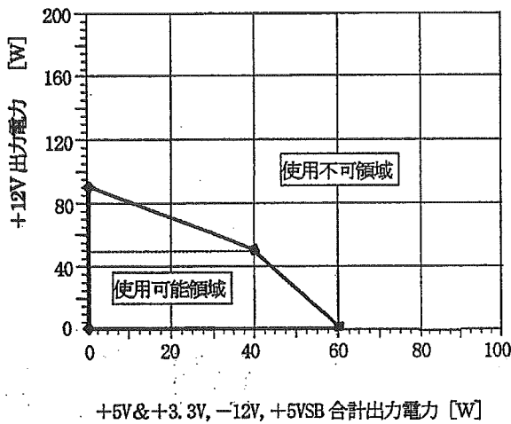
図1. 自然空冷時 (基本構成)
