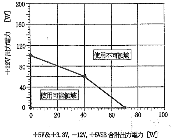
図2. 自然空冷時 (専用アルミ放熱板取付)
