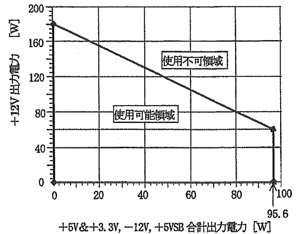
図4. 瞬時定格時 (5秒間以内)
