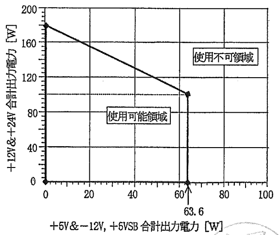
図4. 瞬時定格時 (5秒間以内)
