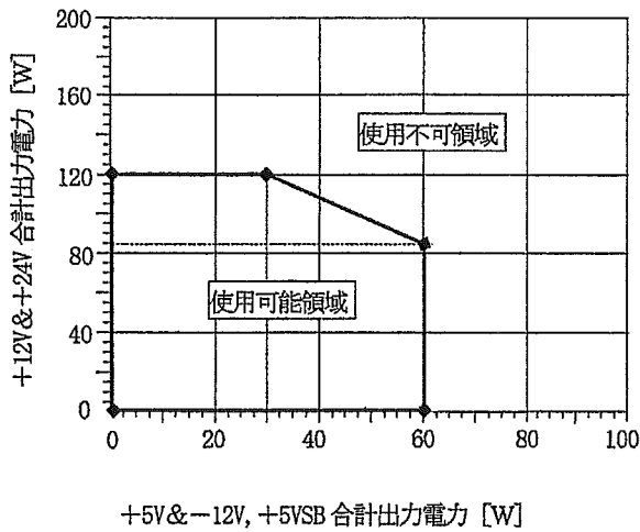
図3. 強制空冷時 (外部ファン使用)
