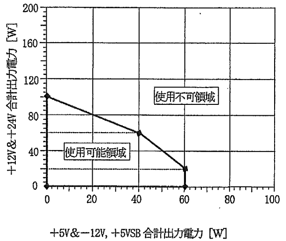
図2. 自然空冷時 (専用アルミ放熱板取付)
