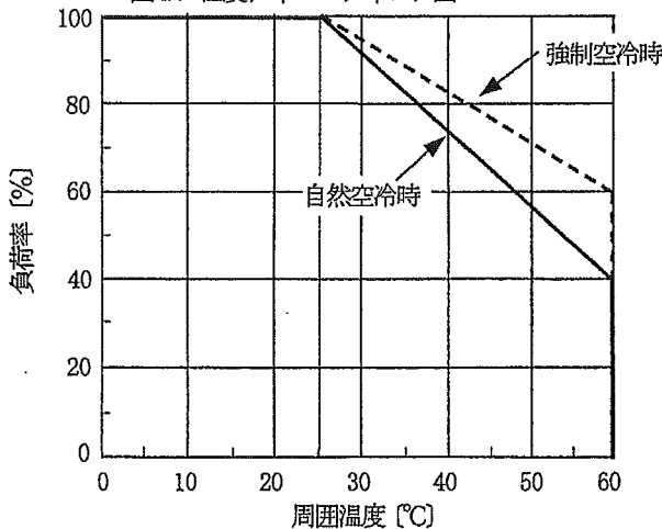
図1. 温度ディレーティング図
