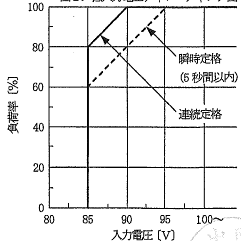
図2. 低入力電圧ディレーティング図
