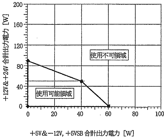
図1. 自然空冷時 (基本構成)
