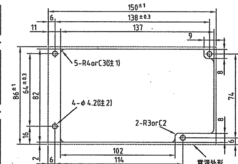
推奨電源取り付け穴加工図
