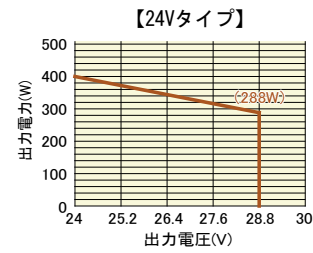
＜図3＞ 設置条件/出力ディレーティング図
