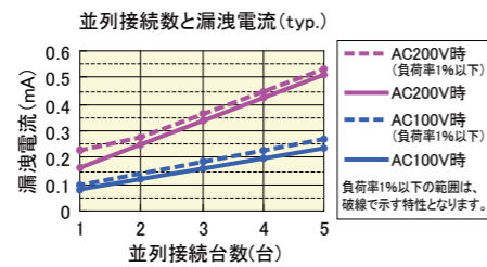
図5 並列接続数と漏洩電流
