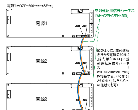
■並列運転用信号ハーネス、接続イメージ図 (電源「mOZP-200-***SE-***」を3台並列接続する場合)
