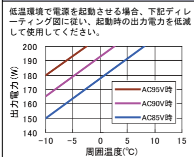
図5 低温環境起動ディレーティング図
