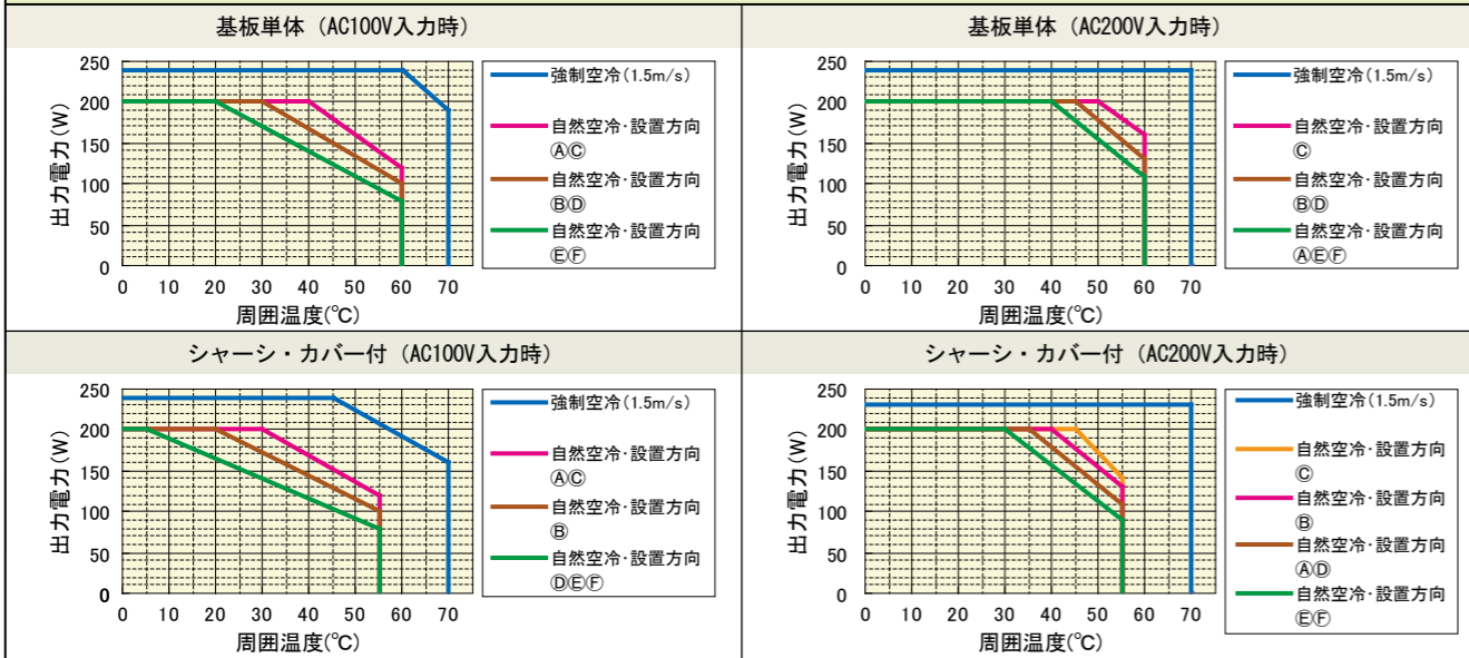
図5 低温環境起動ディレーティング図
