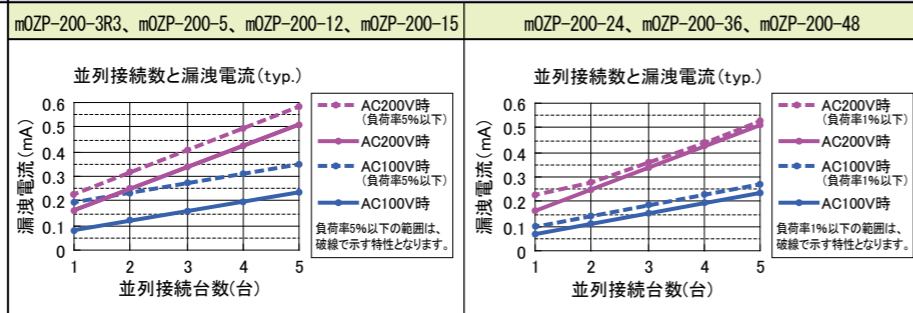
図6 並列接続数と漏洩電流
