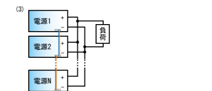
■並列運転用信号ハーネス、接続イメージ図 (電源「mOZP-200-***SE-***」を3台並列接続する場合)
