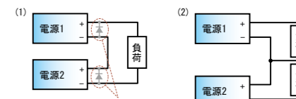
異なる出力電圧の直列接続を行う場合はダイオードを接続してください
