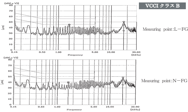
●図8 雑音端子電圧特性 (AC100V 時)
