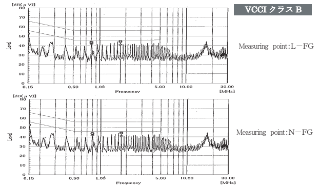
●図9 雑音端子電圧特性 (AC230V 時)
