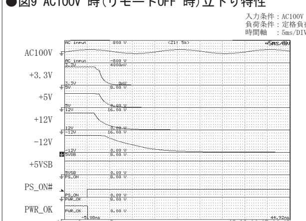
●図9 AC100V 時(リモートOFF 時)立下り特性
