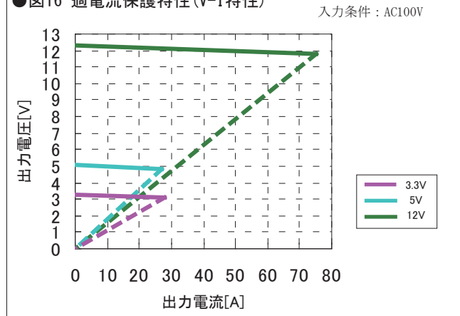
●図16 過電流保護特性(V-I特性)
