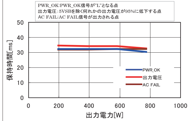
●図12 出力保持時間—出力電力特性
