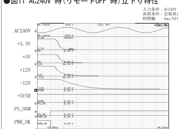
●図11 AC240V 時(リモートOFF 時)立下り特性
