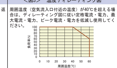
<図3> 温度ディレーティング図
