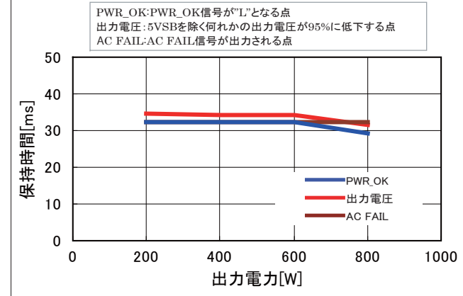
●図25 出力保持時間-出力電力特性
