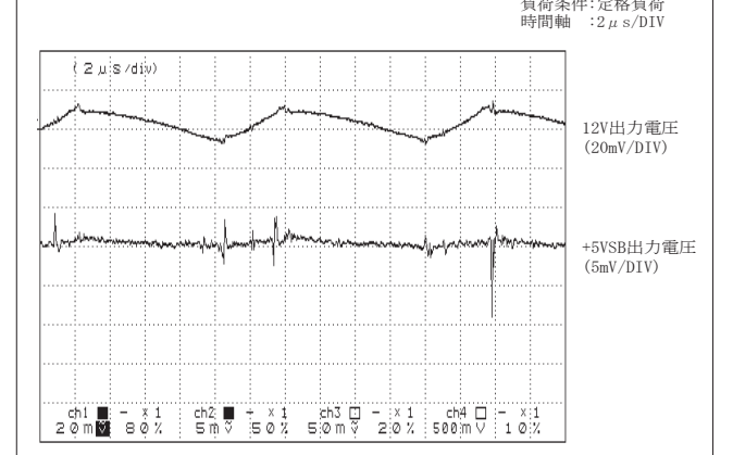
●図28 リップル/スパイク特性
