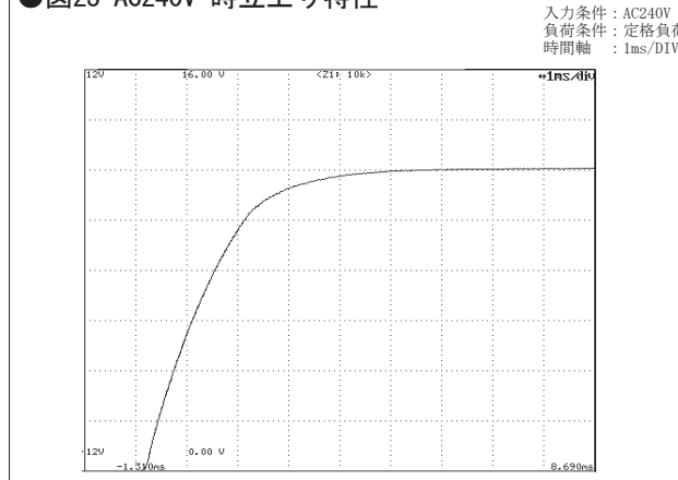
●図23 AC240V 時立上り特性
