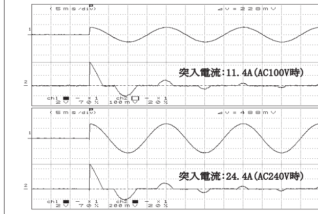
●図19 突入電流特性
