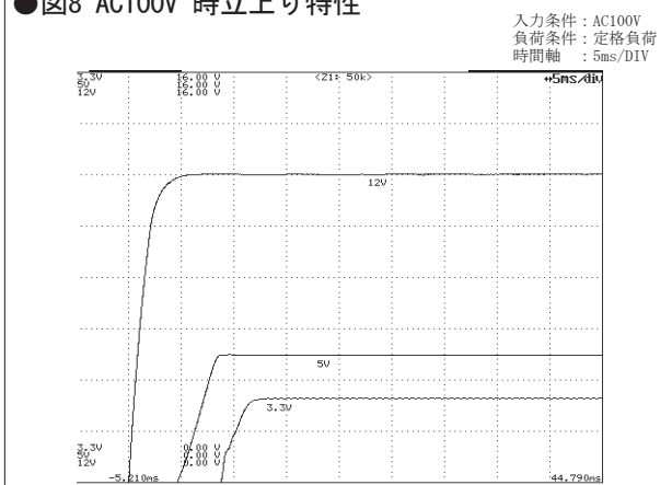
●図8 AC100V 時立上り特性
