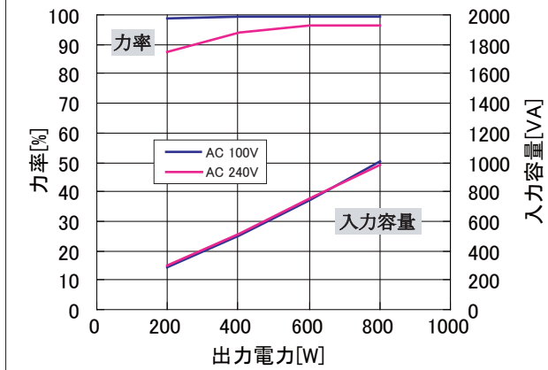
●図18 力率/入力容量-出力電力特性
