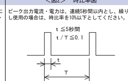
<図2> 時比率図
