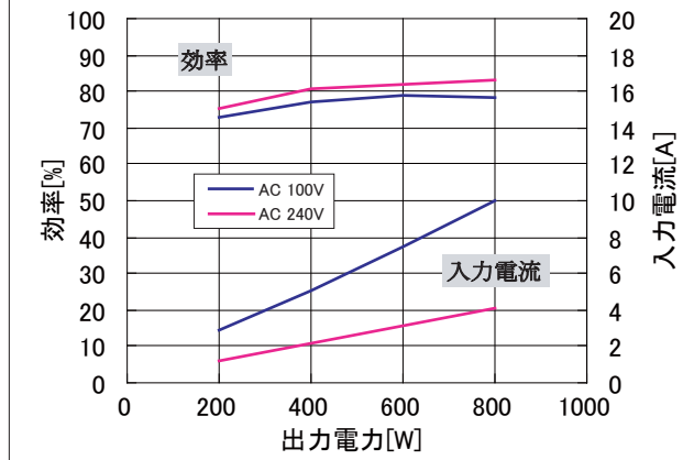
●図17 効率/入力電流-出力電力特性
