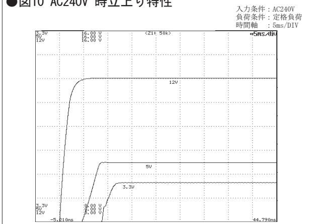
●図10 AC240V 時立上り特性
