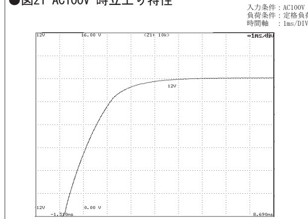
●図21 AC100V 時立上り特性
