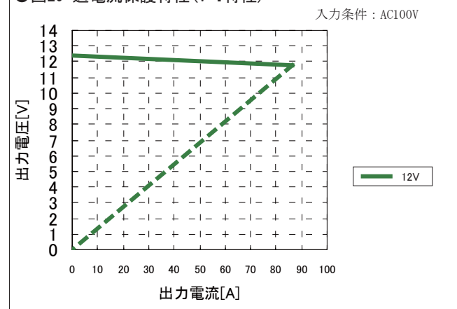
●図29 過電流保護特性(V-I特性)
