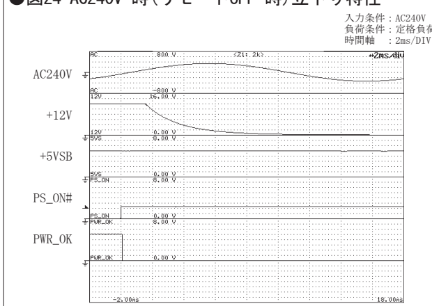
●図24 AC240V 時(リモートOFF 時) 立下り特性
