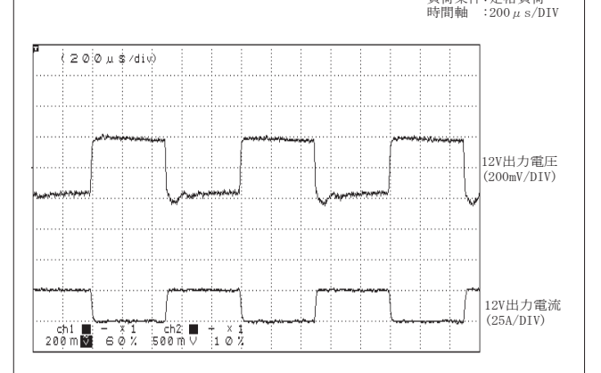
●図26 動的負荷変動特性(1kHz時)
