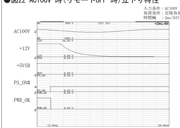
●図22 AC100V 時(リモートOFF 時) 立下り特性
