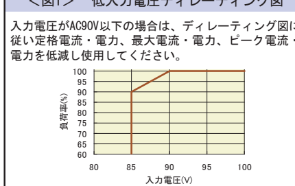
<図1> 低入力電圧ディレーティング図
