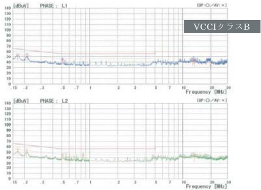
●図8 雑音端子電圧特性 (100V 時)
