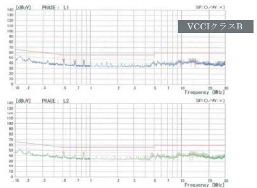
●図9 雑音端子電圧特性 (240V 時)
