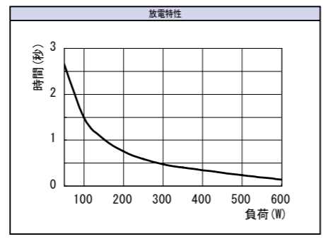
バッテリー充放電特性 (組合せ電源「OZP-350-24-JSE」) (実測の一例) (コンデンサパック使用初期の参考値であり保証値ではありませんのでご注意ください。)
