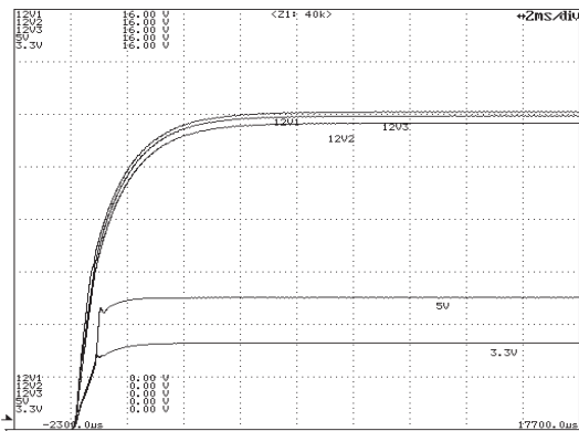
●図10 AC100V 時立上り特性
